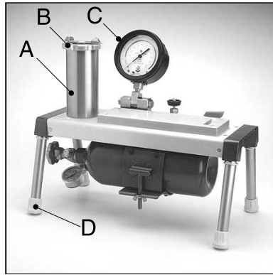
โครงร่าง Plant Water Status Console Consumer รุ่น 3005
