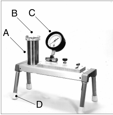
โครงร่าง Plant Water Status Console Consumer รุ่น 3000
