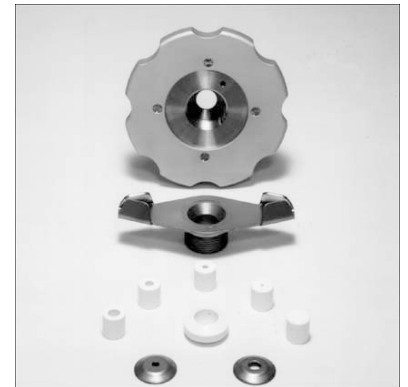
Specimen Holder รุ่น 3015G4 แสดงรูปที่สมบูรณ์พร้อมกับวงแหวนปิดผนึก, sealing sleeves จำนวน 5 อัน และ support washer 2 อัน
